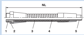
冷卻軟管
