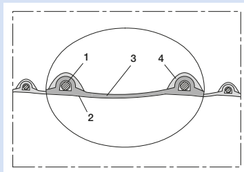
排氣軟管
