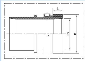
螺紋接頭
