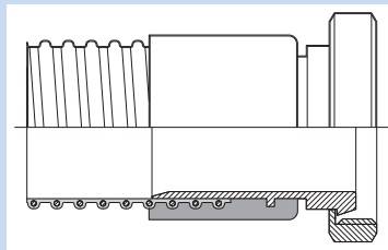
乳品管道配件，依據DIN 2826/11851
