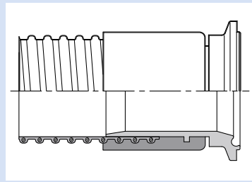
無菌接頭，依據DIN 11864-1 / DIN 11864-3
